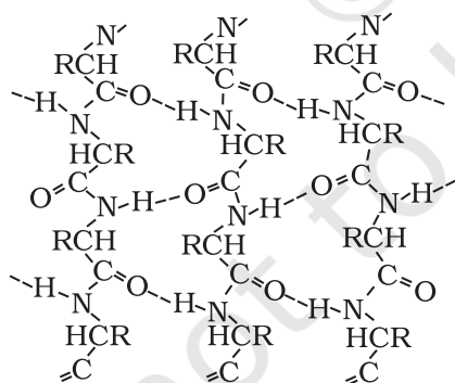
चित्र 10.2— प्रोटीन की \beta -प्लीटेड शीट संरचना
