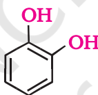
सामान्य नाम आईयूपीएसी नाम कैटेकोल बेन्जीन 1, 2- डाइऑल
