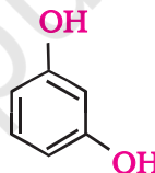
रिसॉर्सिनॉल बेन्जीन 1, 3- डाइऑल
