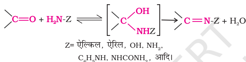
सारणी 8.2- ऐल्डिहाइडों व कीटोनों ( >\text{C}=\text{N}-\text{Z} ) के कुछ N- प्रतिस्थापित व्युत्पन्न
