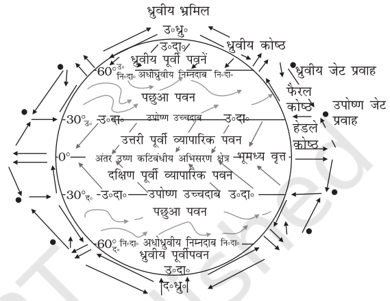
चित्र 9.6 : वायुमंडल का सरलतम सामान्य परिसंचरण
