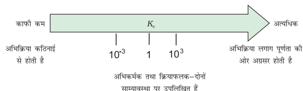
चित्र 6.6 K_c पर अभिक्रिया की सीमा का निर्धार करना
