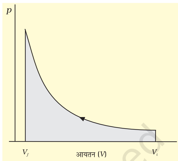
चित्र 5.5 (ग) pV वक्र जब प्रारंभिक आयतन V_i से V_f तक पहुँचने के लिए उत्क्रमणीय परिस्थितियों में लगातार बदलते हुए अस्थिर दाब पर अनंत पदों में किया गया कार्य छायादार क्षेत्र से दर्शाया गया है।
