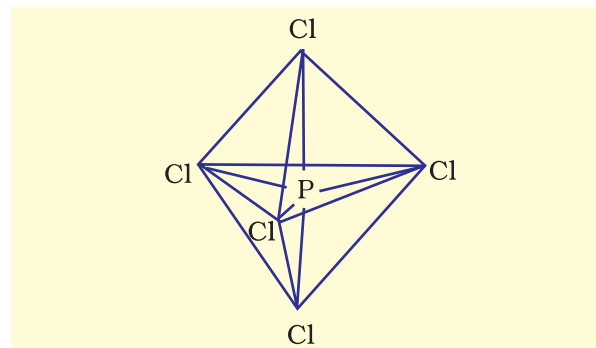
चित्र 4.17 PCl_5 अणु की त्रिकोणीय द्वि-पिरामिडी ज्यामिति
