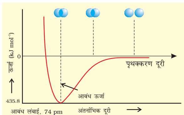
चित्र 4.8: H_2 अणु के विरचन के लिए H परमाणुओं के बीच अंतराणाधिक दूरी की सापेक्ष स्थितिज ऊर्जा का आरेख, आरेख में न्यूनतम ऊर्जा स्थिति H_2 की सर्वाधिक स्थायी अवस्था दर्शाती है।
